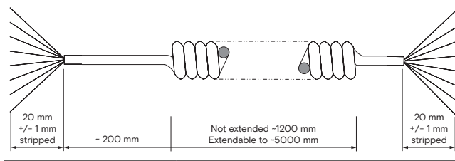
Cable - H1200-5000 (1000457)
