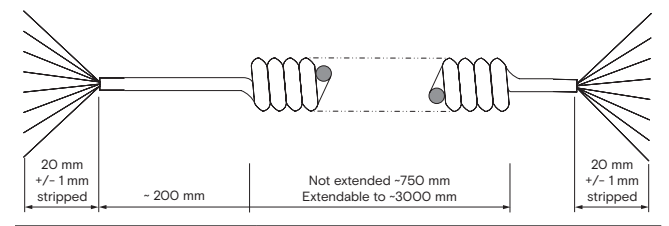
Cable - H750-3000 (1000458)
