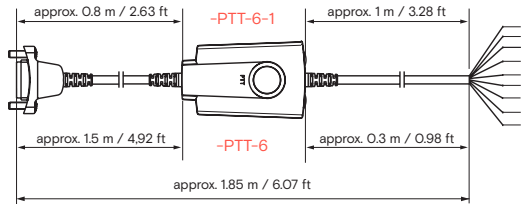
Cable PTT-6 (500844) Cable PTT-6-1 (502418)
