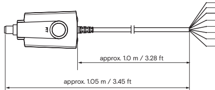
Cable - PTT 32 C6 (1000373)
