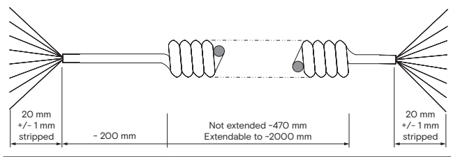
Cable - H470-2000 (1000456)
